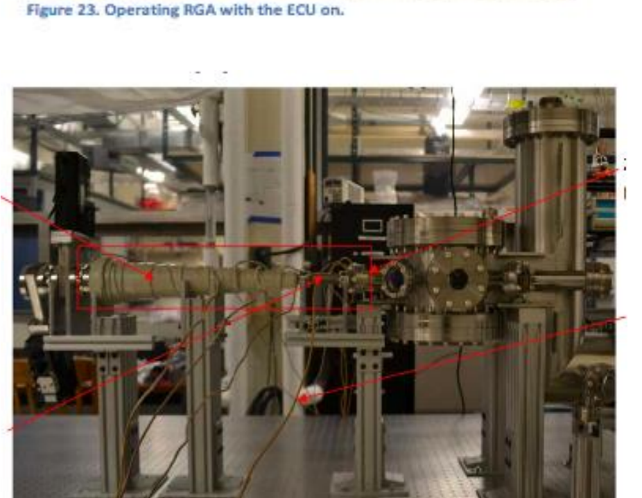
(*) Sistema de vacío para átomos ultra-fríos diseñado y construido en MIT (USA)
